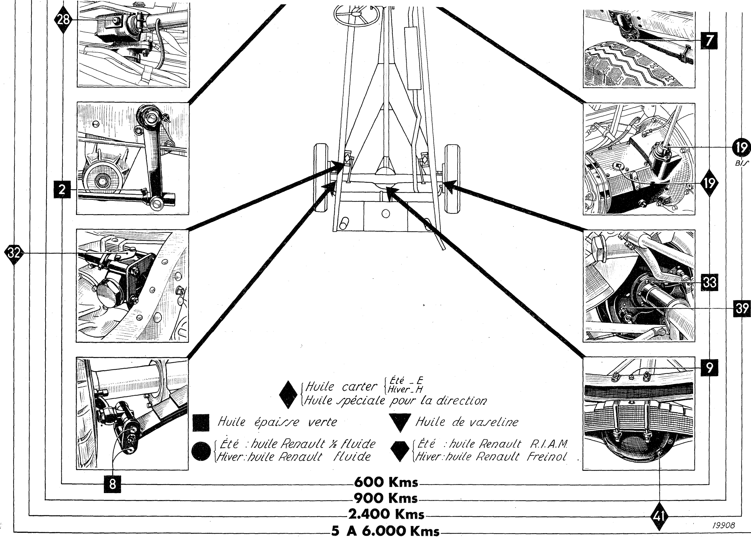
Fig. 4. — SCHÉMA DE GRAISSAGE.
